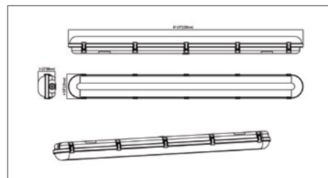
4117WH-3W-3CCT-MS-EM_Main.jpg
