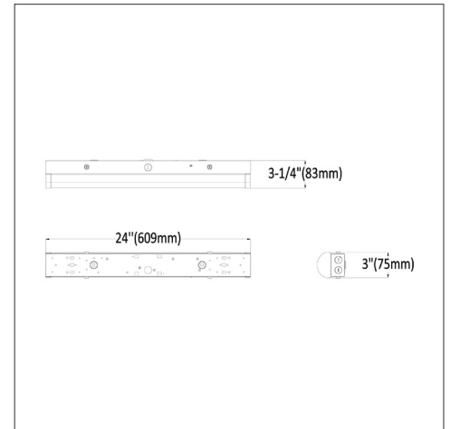
4125WH-3W-3CCT-MS-EM_Main.jpg
